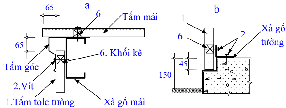
a . Liên kết tường với mái
