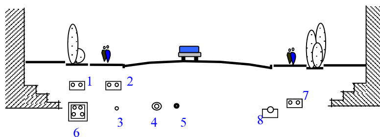
P/a Bố trí phân tán
