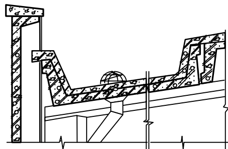
Giải pháp thoát nước Sênô
