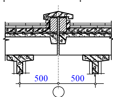
Chống dột tại khe biến dạng
