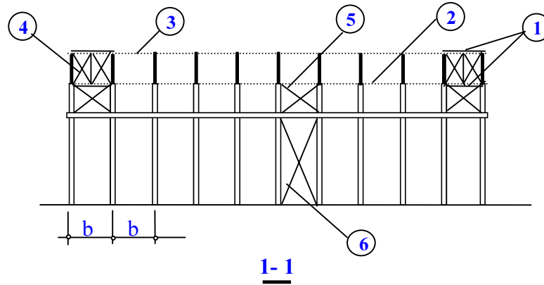
Hệ thống giằng đứng kết cấu mang lực mái và giằng cột
