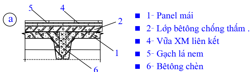
a - MÁI KHÔNG CÁCH NHIỆT VN
