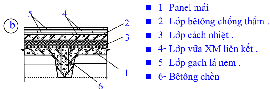
b - MÁI CÓ CÁCH NHIỆT VN
