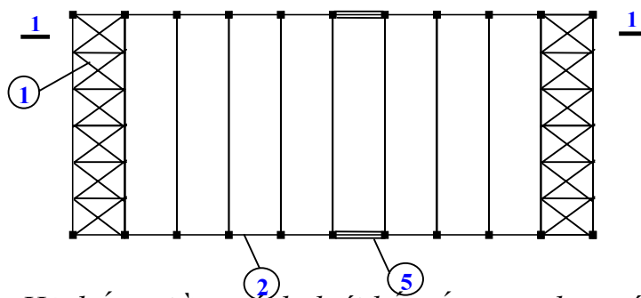
Hệ thống giằng cánh dưới kết cấu mang lực mái
